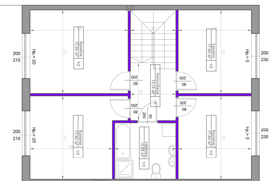
PIĘTRO
